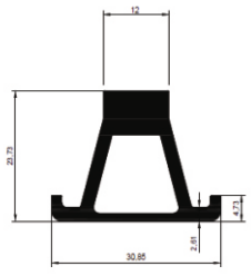
Alüminyum Özel Somun Aluminum Special Nut
