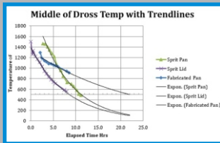
Cooling curves 冷却时间的比较
