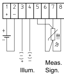
Type -PxL4, -PTxL4 (4-wire)
